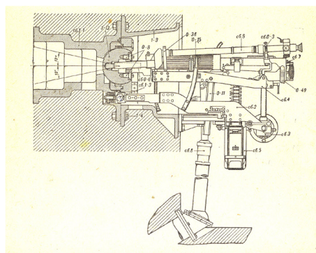
Установка НПС-3 [24].
