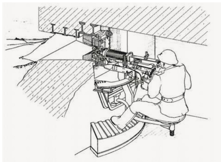
Установка ПСК-2 [12].
