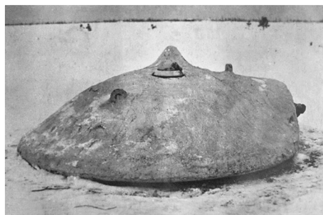
Пулеметная бронебашня ВПФС (К-6) [12].
