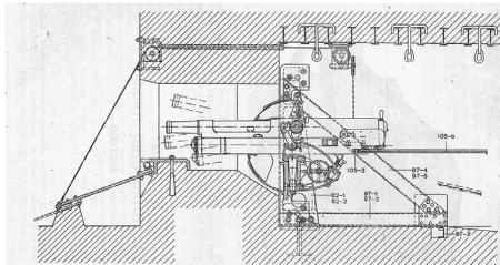
Казематная 76-мм установка 1932 года [19].
