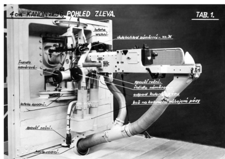
Чехословацкая установка для 47-мм пушки спаренной с 7,92-мм пулеметом [25].
