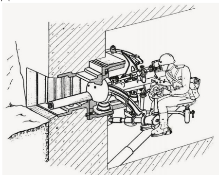
Казематная артиллерийская установка с 76-мм пушкой ДОТ-2 [12].
