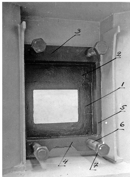
Амбразурные детали ПСК-2, вид из каземата:
