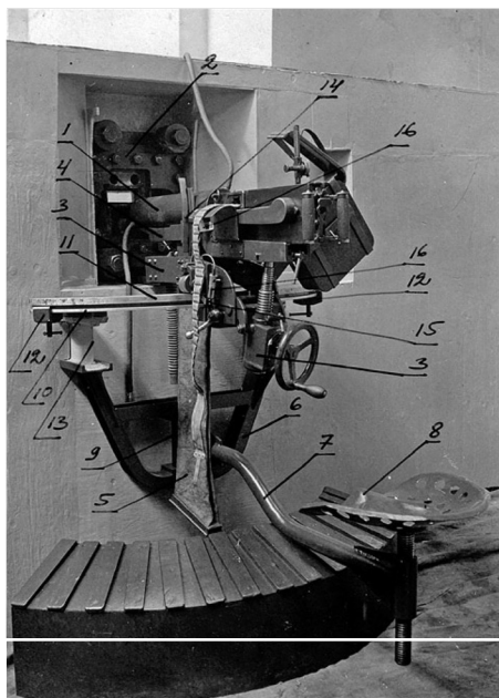
Казематная пулеметная установка ПСК-2 на стенде:
