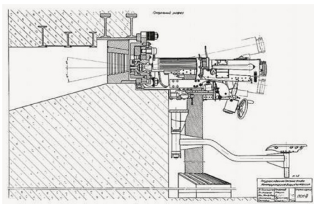
Пулеметный станок ПСК-2 [12].
