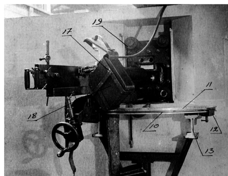
Установка ПСК-2 на стенде, вид справа: 10 - опорный сектор; 11 - шкала горизонтального наведения; 12 - ограничитель; 13 консольная балка; 17 - корзина; 18 - коробка; 19 - пружины Бельвиля [16].
