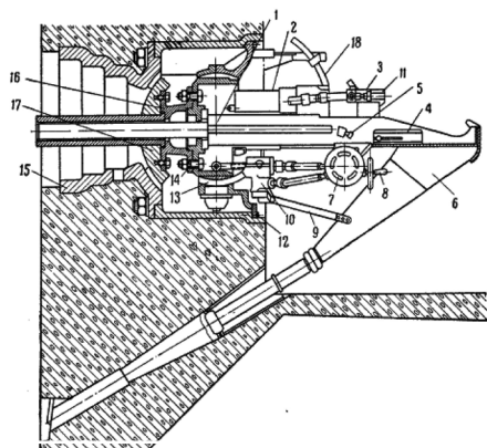
Артиллерийская установка Л-17 образца 1940 года:
