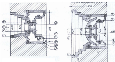
Артиллерийская установка Л-17.
