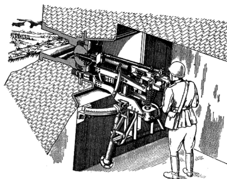
Установка НПС-3 [12].
