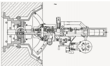
Установка ДОТ-4. План [12].
