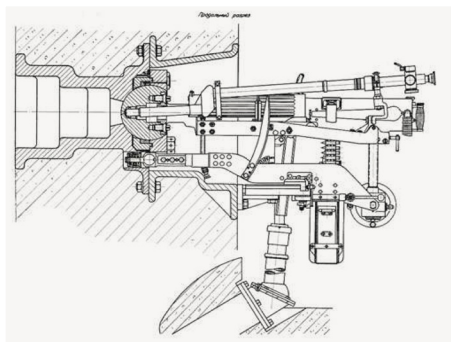
Пулеметный станок НПС-3 [12].
