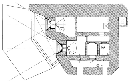
Общий вид артиллерийского полукапонира 1938 года [15].
