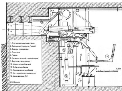
Пулеметный станок ПС-31 В.П. Горносталева [18].
