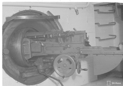
Установка Л-17 в финской огневой точке [22].
