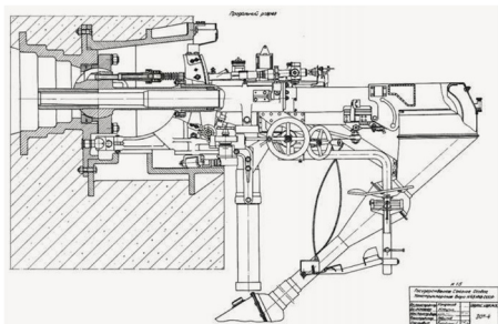
Установка ДОТ-4 [12].
