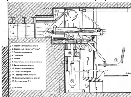
Пулеметный станок ПС-31 Горностаева [18].
