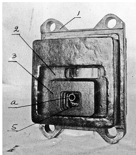
Амбразурные детали ПСК-2, вид с поля: 1 - корпус заслонки; 2 - бронеплита; 3 - щиток подвижной; 5 - шар; а - сосок шара [16].
