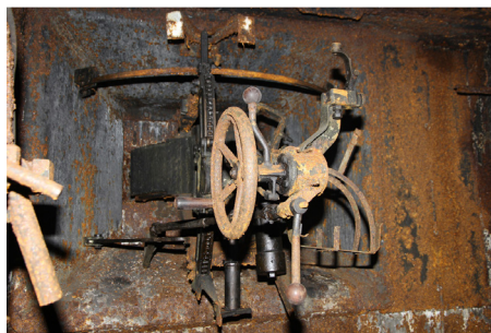
Установка КПУ (И-10) [17].
