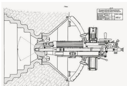
Пулеметный станок НПС-3. План [12].
