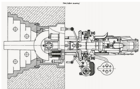
Казематная артиллерийская установка с 76-мм пушкой ДДТ-2. План [12].
