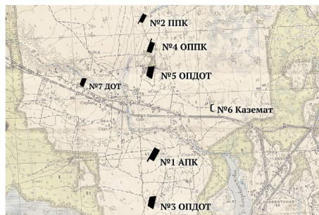
Схема расположения опытных сооружений в районе Охта.
