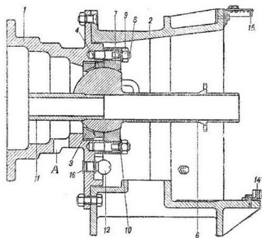
Элементы установки ДОТ-4.
