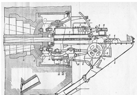
Установка Л-17 [21].
