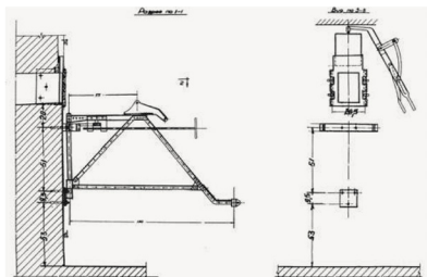
Пулеметный станок Юшина [12].
