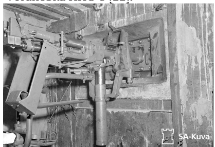
Установка ДОТ-4 [22].
