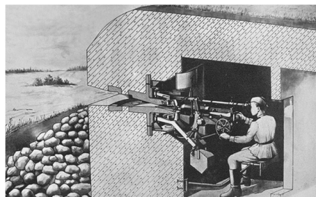
Установка КПУ (И-10) [12].
