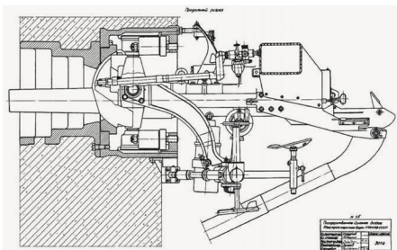
Казематная артиллерийская установка с 76-мм пушкой ДОТ-2 [12].
