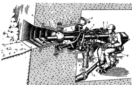
Установка ДОТ-4.
